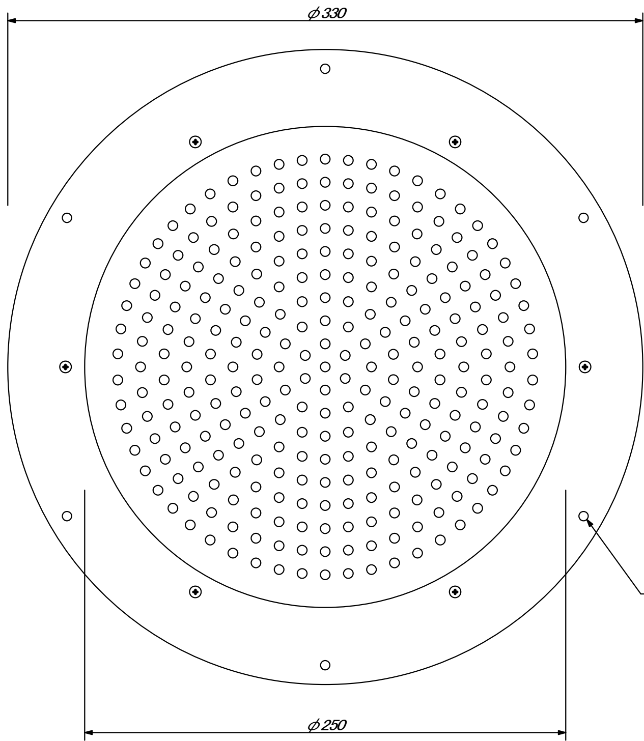
\phi 5 LED271個
